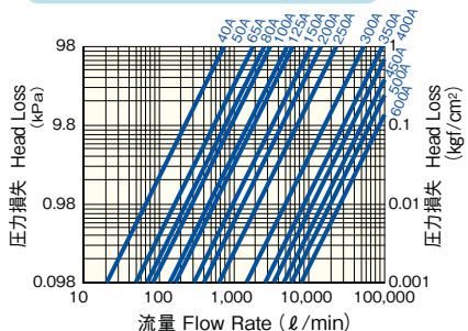
バタフライバルブ Butterfly Valve
