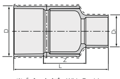
※プッシュタイプ With Bushing
